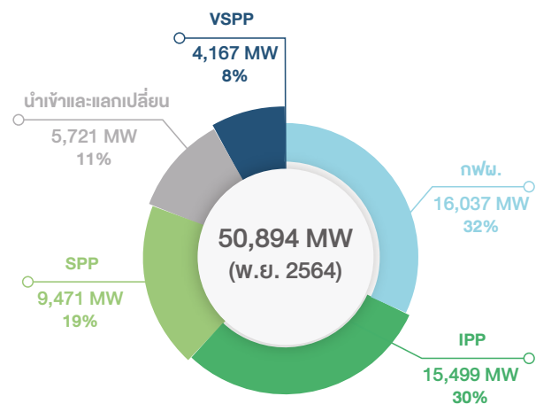
กำลังผลิตตามสัญญาในระบบไฟฟ้า ณ สิ้นเดือนพฤศจิกายน 2564
