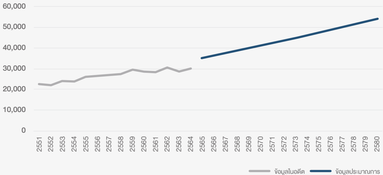
กราฟแสดงความต้องการใช้ไฟฟ้าสูงสุดในประเทศไทยปี 2551-2580 (เมกะวัตต์)
